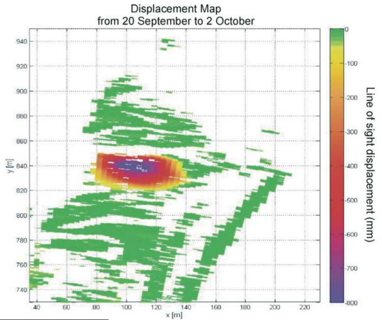
Fig.13 - Esempio di mappa cromatica degli spostamenti lungo la linea di vista misurati dell'interferometro. Dati registrati tra le 00:01 del 20 settembre e le 11:31 del 2 Ottobre. Tali valori corrispondono a spostamenti in avvicinamento al radar - Example of colour map of displacements along the line of sight measured by the interferometer. Data recorded from 00:01 of 20 September to 11:31 of 2 October. These values correspond to displacements approaching the radar
