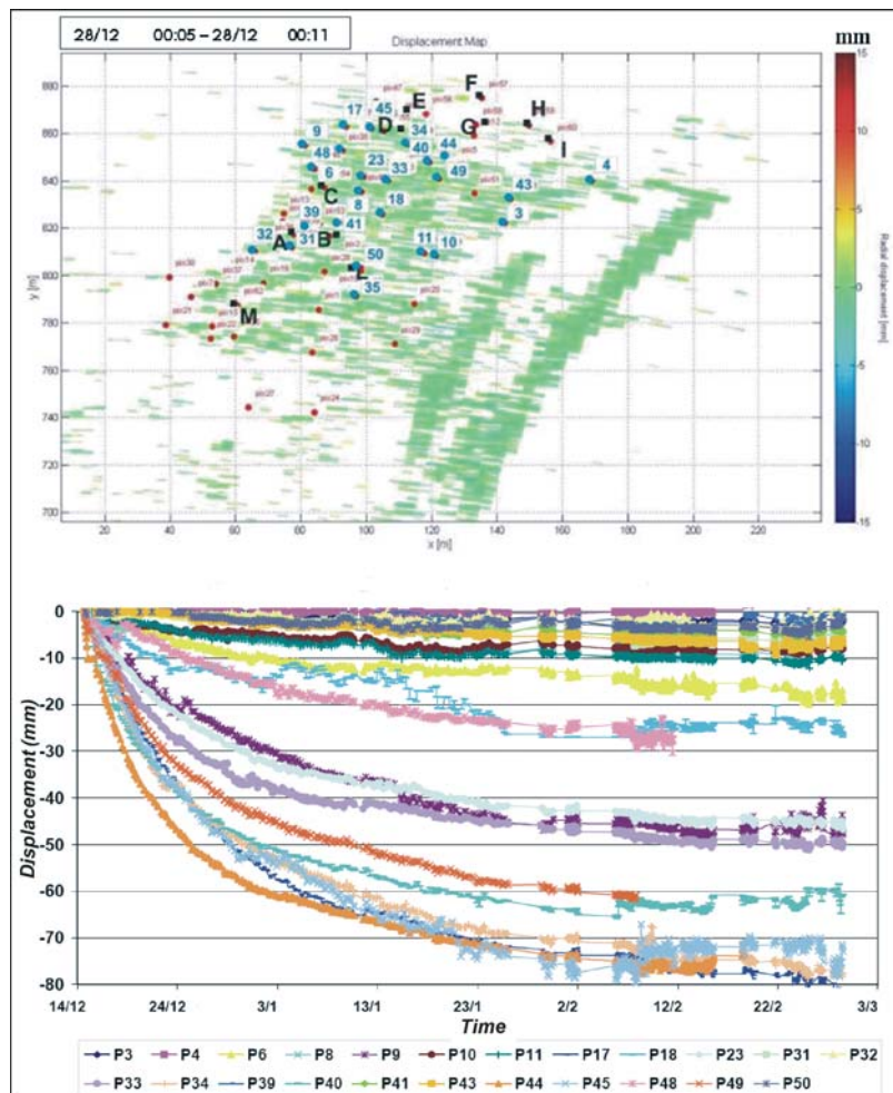
Fig.14 - Serie temporali degli spostamenti di alcuni pixel registrati tra il 14 Dicembre ed il 29 Febbraio. L'ubicazione dei punti è riportata nella figura in alto - Time series of displacements of some pixels recorded from 14 December to 29 February. The location of the points is shown in the top figure
