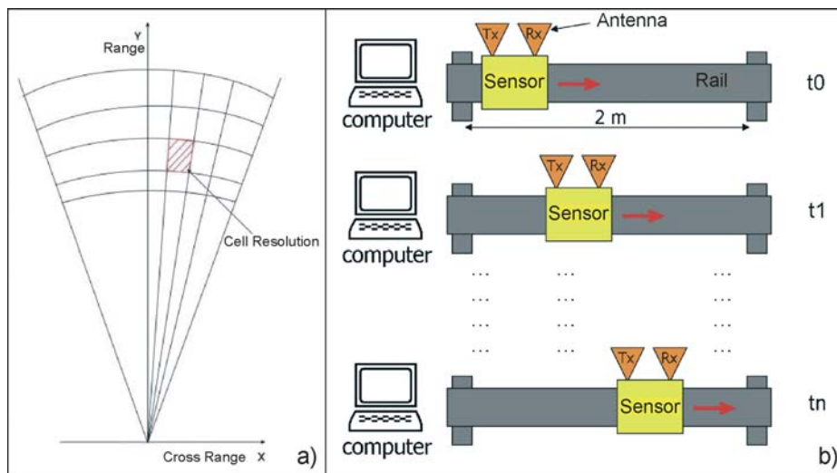
Fig.1 - a) Griglia di acquisizione dell'immagine SAR; b) Schema di funzionamento dell'interferometro SAR terrestre - SAR image acquisition grid; b) Schematic diagram of ground-based SAR interferometer
