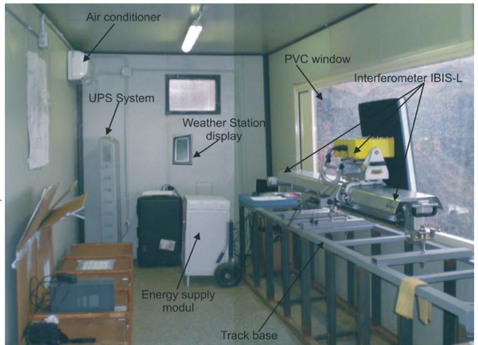
Fig.4 - Vista dell'interno del box e dei vari apparecchi che costituiscono il sistema di monitoraggio - View of the interior of the box and of the various components of the monitoring system
