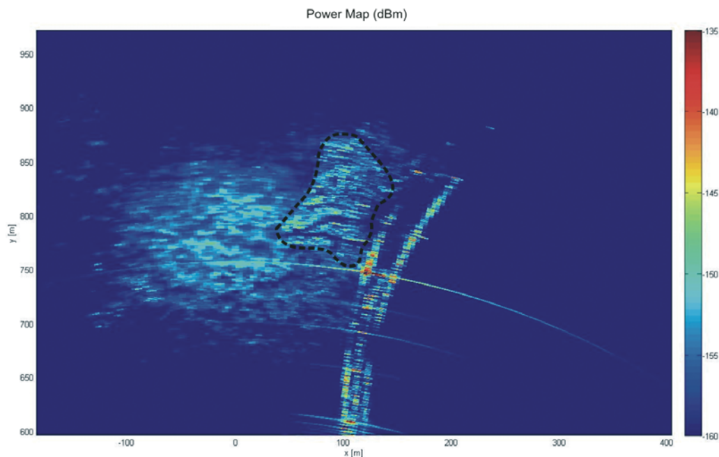
Fig.9 - Mappa in potenza dello scenario irradiato. La linea nera tratteggiata identifica il settore di versante privo di vegetazione mostrato in Fig.2 - Power map of the scanned scenario. The dashed black line identifies the unvegetated slope sector of Fig. 2
