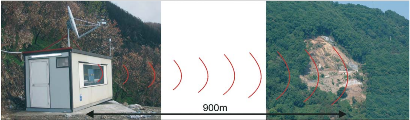
Fig.2 - Schema operativo con foto della piattaforma di monitoraggio e del versante affetto da condizioni di instabilità - Schematic diagram of the system with photo of the monitoring platform and of the unstable slope
