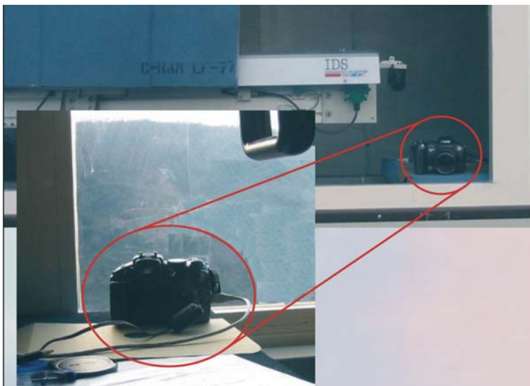
Fig.7 - Fotocamera con acquisizione automatica - Automatic photo camera
