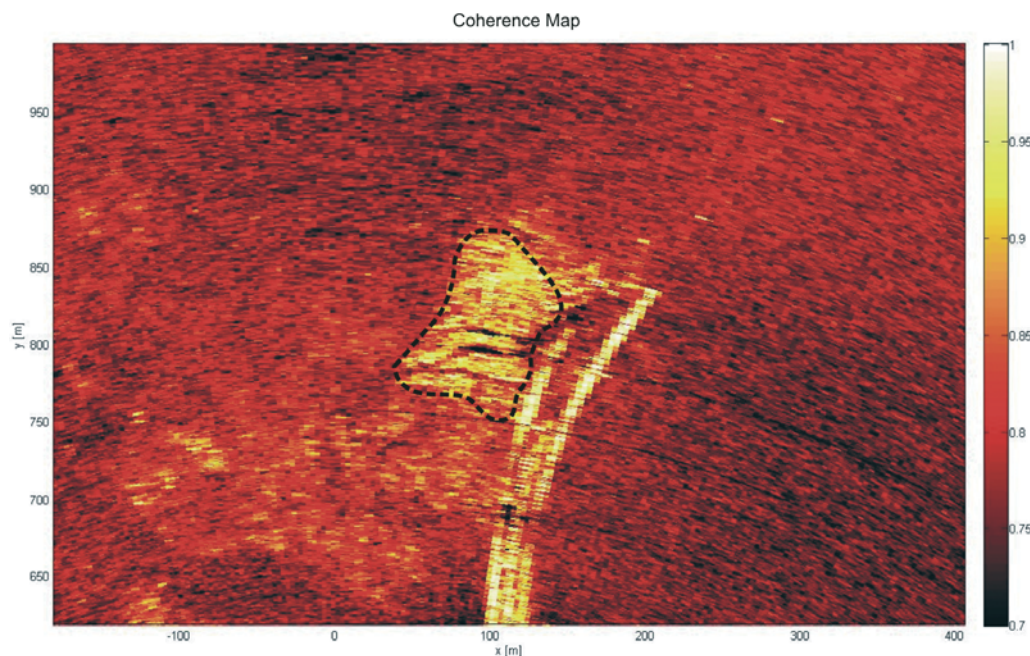
Fig. 10 - Mappa di coerenza dello scenario irradiato. La linea nera tratteggiata identifica il settore di versante privo di vegetazione mostrato in Fig.2 - Coherence map of the scanned scenario. The dashed black line identifies the unvegetated slope sector of Fig.2
