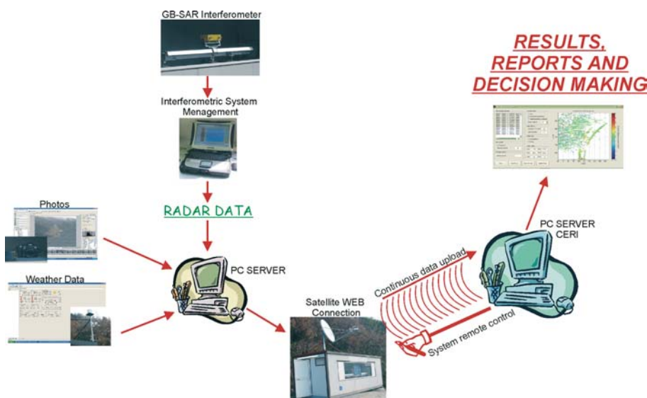
Fig.8 - Diagramma di flusso che descrive l'intera architettura del sistema di monitoraggio dall'acquisizione dati sino alla creazione di report informativi - Flow diagram describing the complete architecture of the monitoring system, from acquisition to reporting of the data
